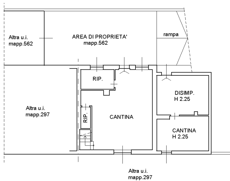
PIANO PRIMO INTERRATO (S1) H 2,40 m
